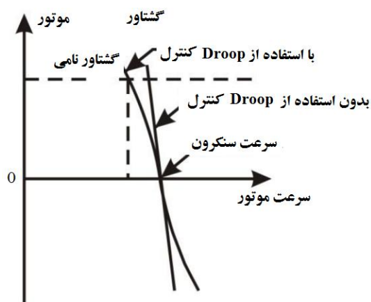
شکل ۶-۲۱ نمودار کنترل افتادگی
