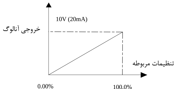
شکل ۱۴-۶ رابطه بین AO و تنظیمات مربوطه
